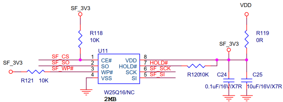
图 1-10 Nor Flash 原理图
