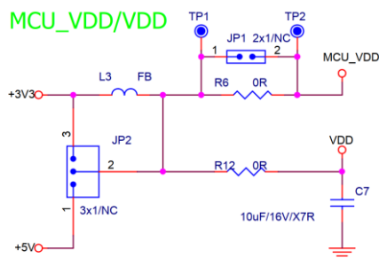
图 1-8 供电切换电路图
