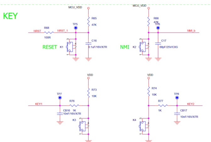
图 1-13 Reset/NMI/key 电路图
