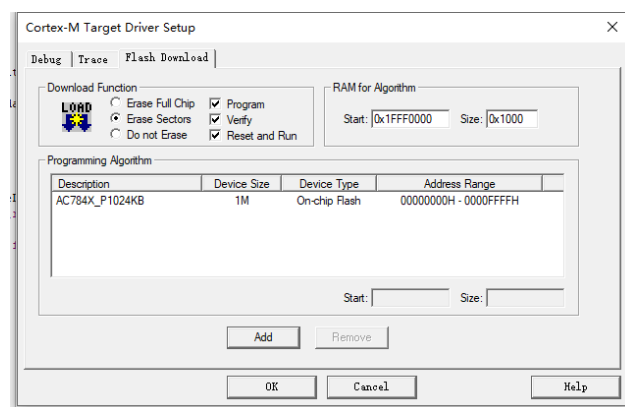
图 3-11 Flash Download 选项卡设置
