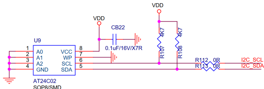
图 1-11 EEPROM 原理图
