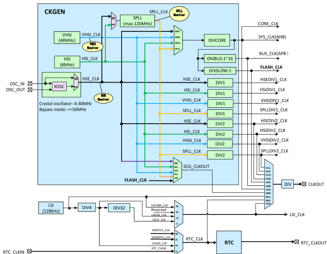
图 4-2 时钟树
