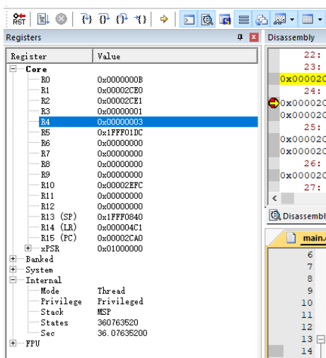
图 3-19 查看 CPU
