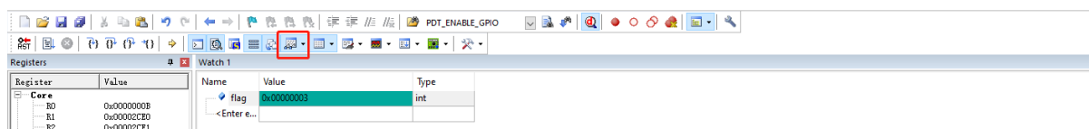
图 3-16 变量监控
