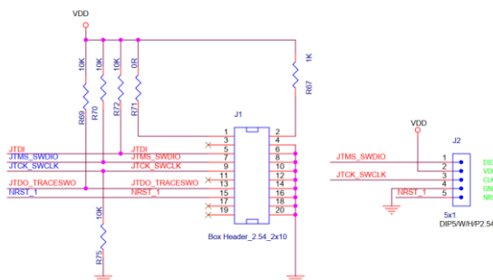
图 1-12 调试接口
