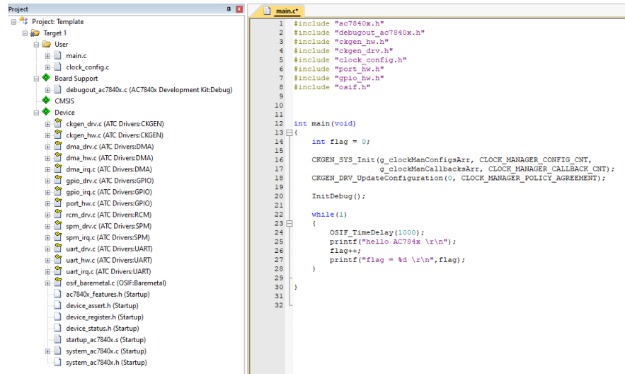
图 3-7 输出代码
