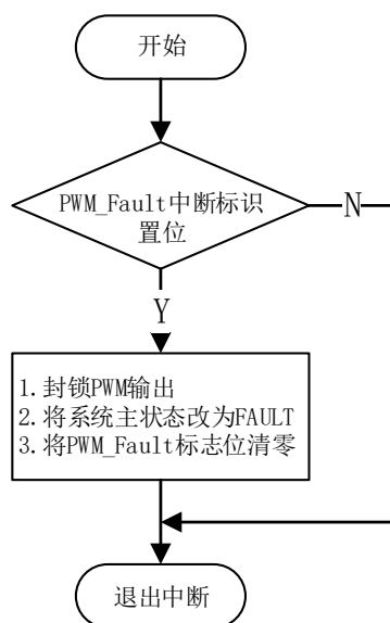
图 3-1 硬件过流中断服务程序
