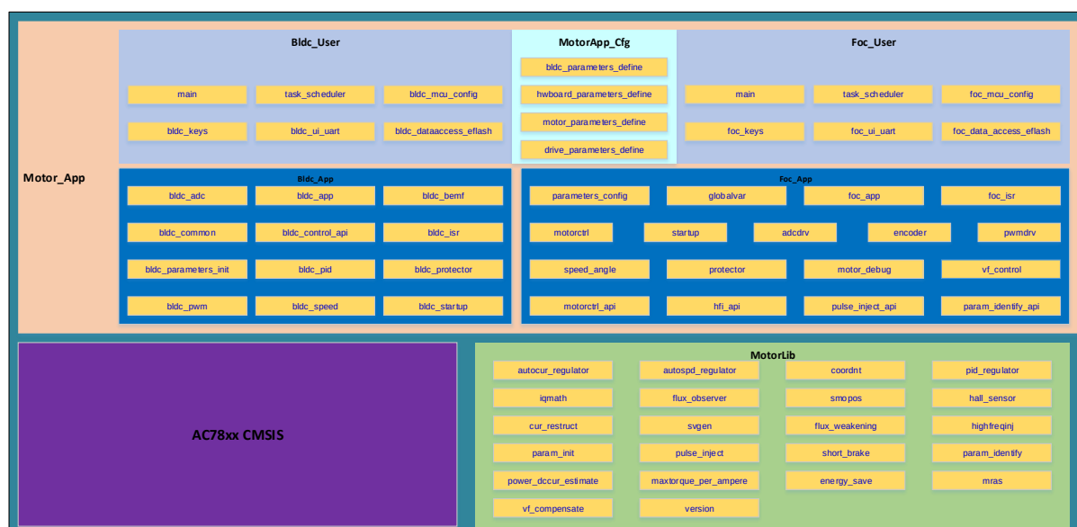
图 1-3 Motor_App 架构图
