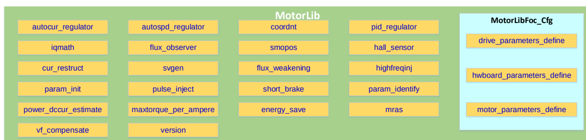
图 2-1 MotorLib 架构图
