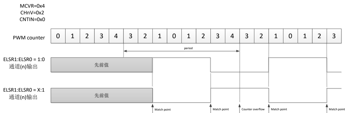
图 11-9 CPWM 波形
