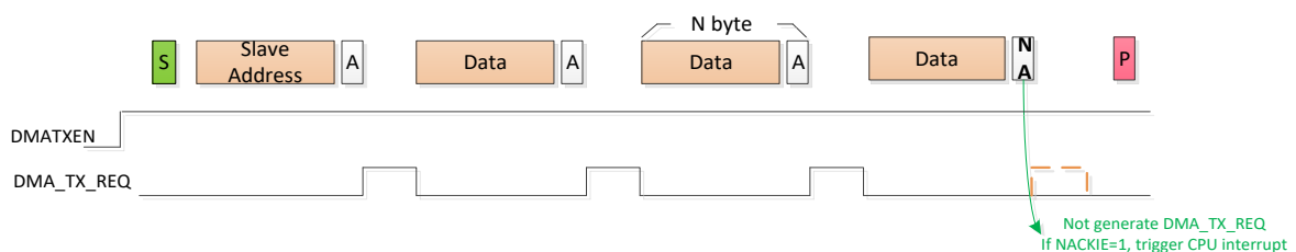
图 17-11 从机发送器
