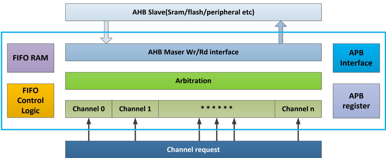
图 19-1 DMA 结构框图
