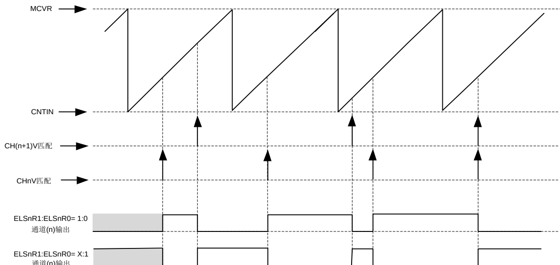
图 11-24 CH(n+1)V 在下一周期匹配的输出生波形
