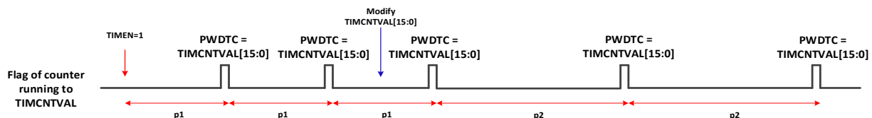
图 12-9 TIMEN=1 期间修改 TIMLDVAL
