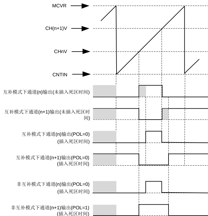
图 11-23 死区时间插入
