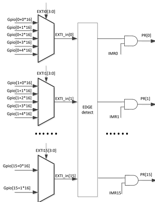
图 16-2 GPIO 外部中断
