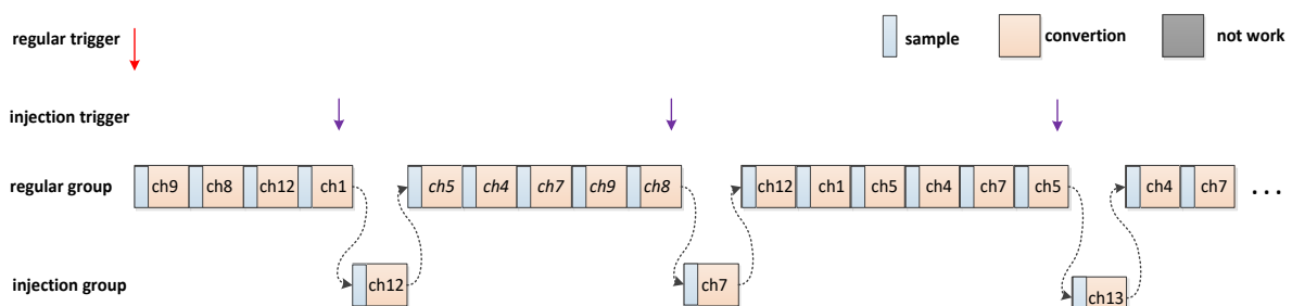
图 9-15 Mode 5 注入组间隔模式工作流程
