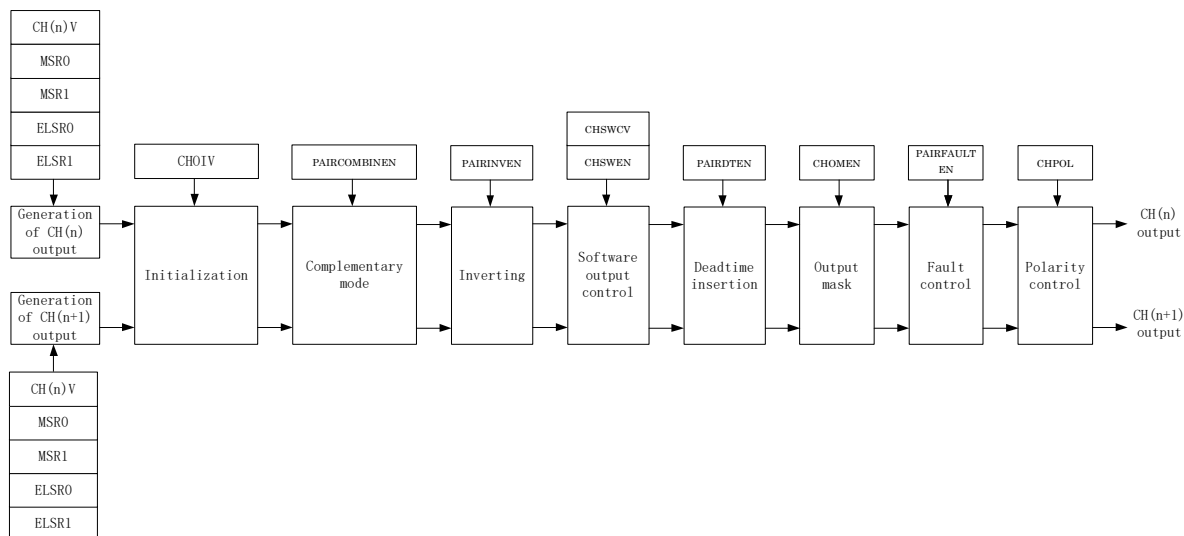
图 11-40 特性优先级
