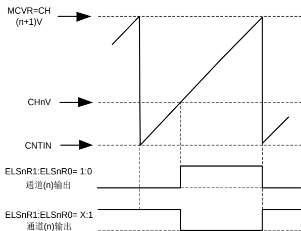
图 11-12 (CNTIN < CHnV < MCVR) & (CH(n+1)V = MCVR)条件下输出波形
