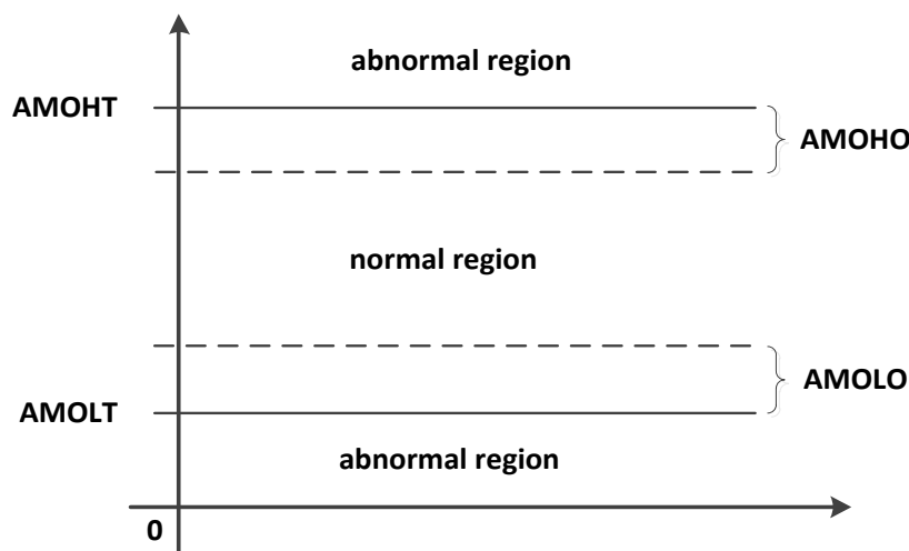
图 9-20 边沿触发模式下监控区域
