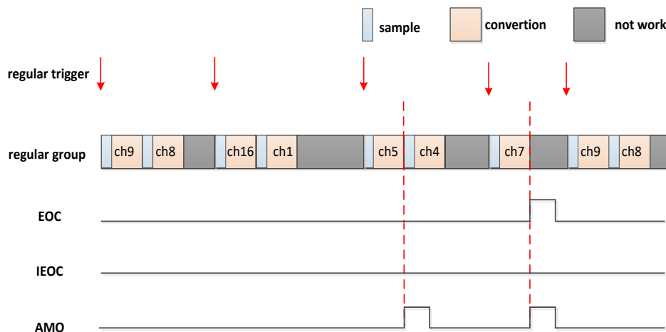
图 9-22 情形 2 下的三个标志行为
