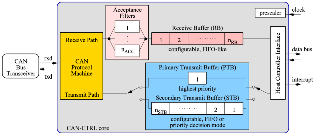
图 7-2 消息缓冲区示意图
