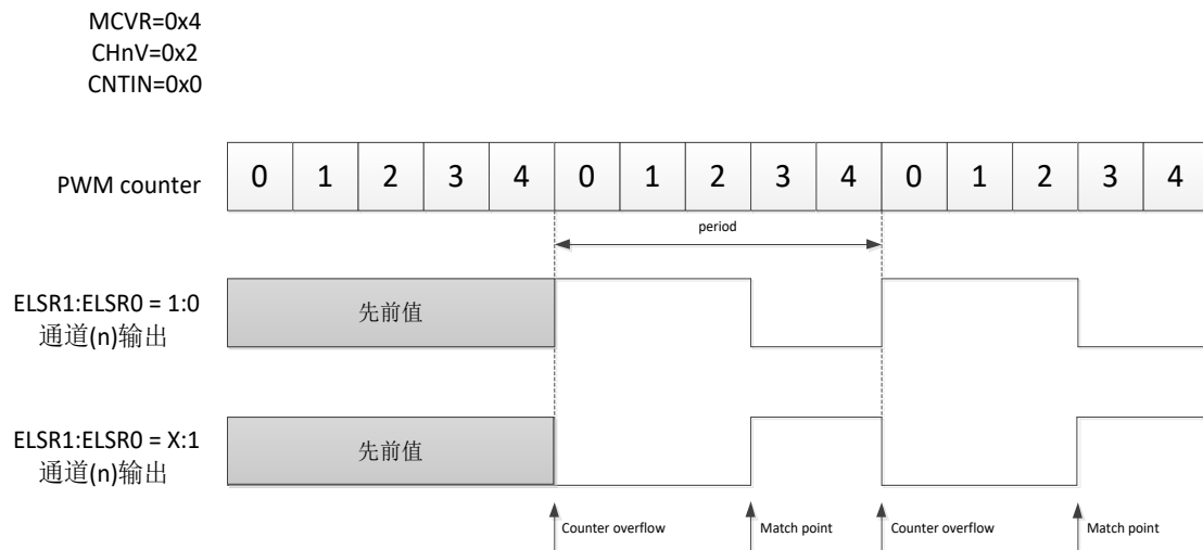
图 11-8 EPWM 波形
