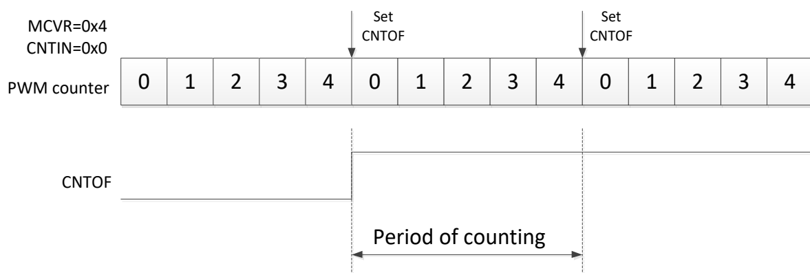
图 11-2 向上计数
