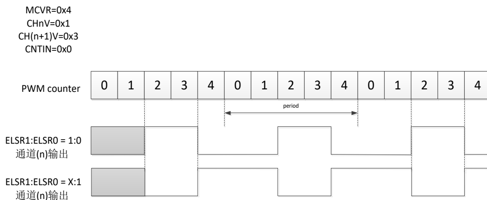
图 11-10 向上计数组合模式输出波形
