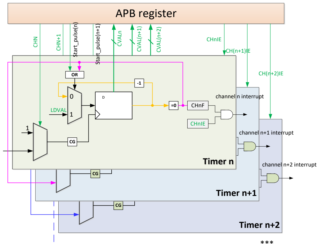
图 13-1 TIMER 结构框图
