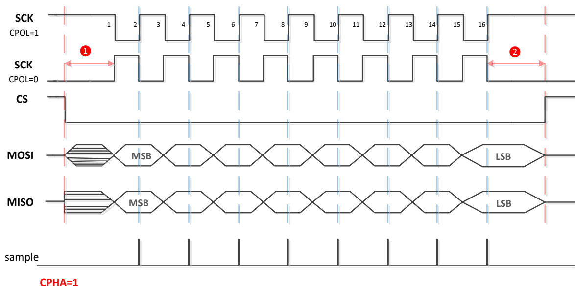
图 18-6 CPHA=1 传输格式
