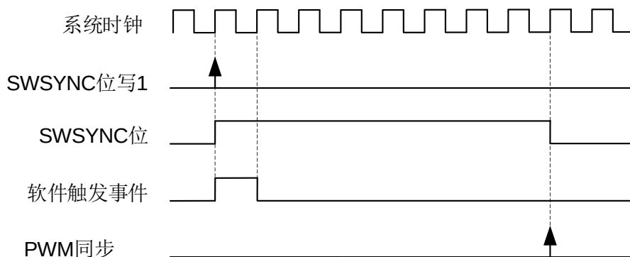
图 11-32 软件触发事件
