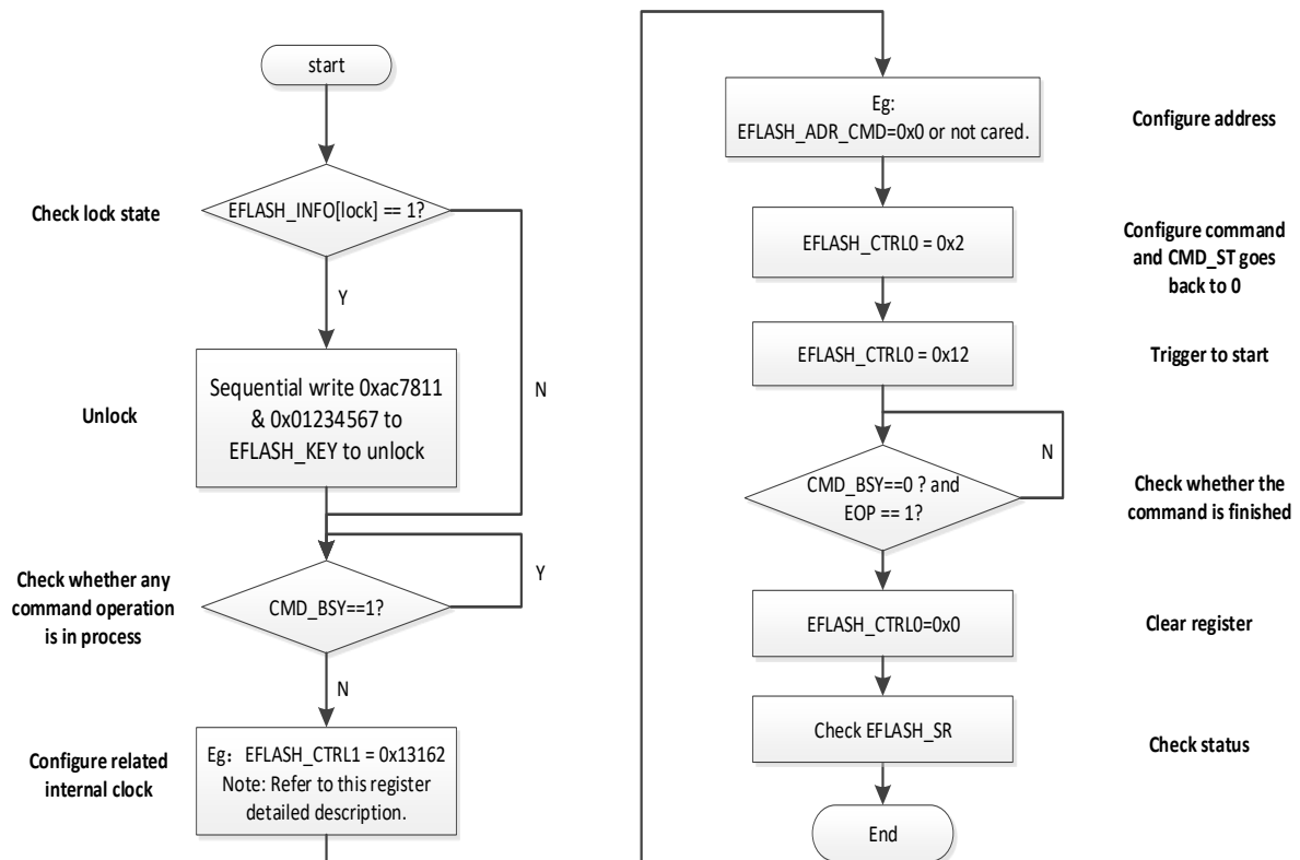
图 22-4 整片擦除命令操作流程
