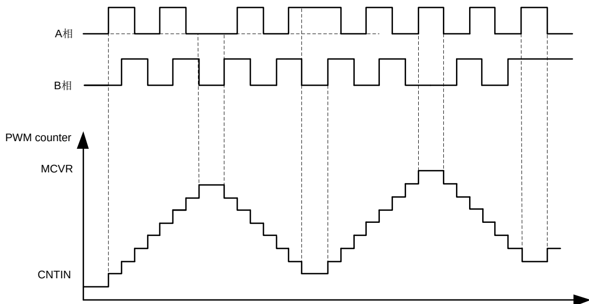
图 11-28 A 相和 B 相编码模式
