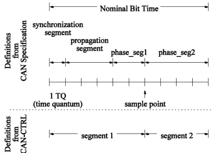
图 7-5 CAN 位定时
