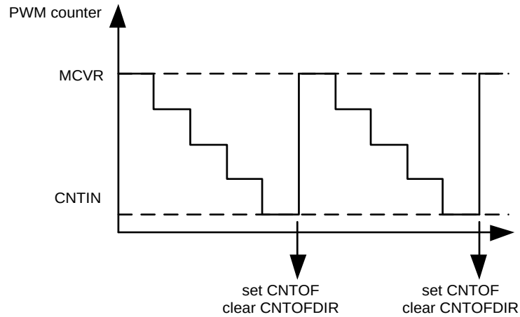
图 11-30 向下计数 PWM counter 溢出
