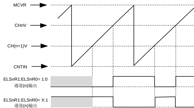
图 11-14 (CNTIN < CH_nV / CH_{(n+1)}V < MCVR) 且 (CH_nV > CH_{(n+1)}V) 条件下输出波形
